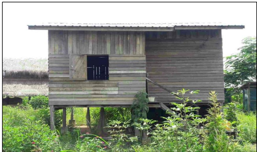
စစ်ကိုင်းတိုင်းဒေသကြီး၊ ကလေးမြို့နယ်ရှိ ပြောင်းရွှေ့နေအိမ်များ တည်ဆောက်ခြင်းလုပ်ငန်း ဆောင်ရွက်ပြီးစီးမှုမှတ်တမ်းဓာတ်ပုံ
